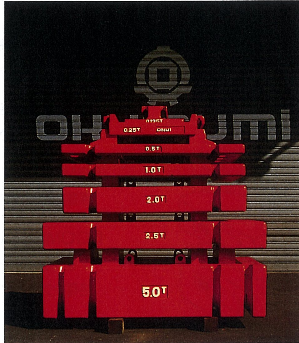
0.125~5.0t 組み合わせ写真
