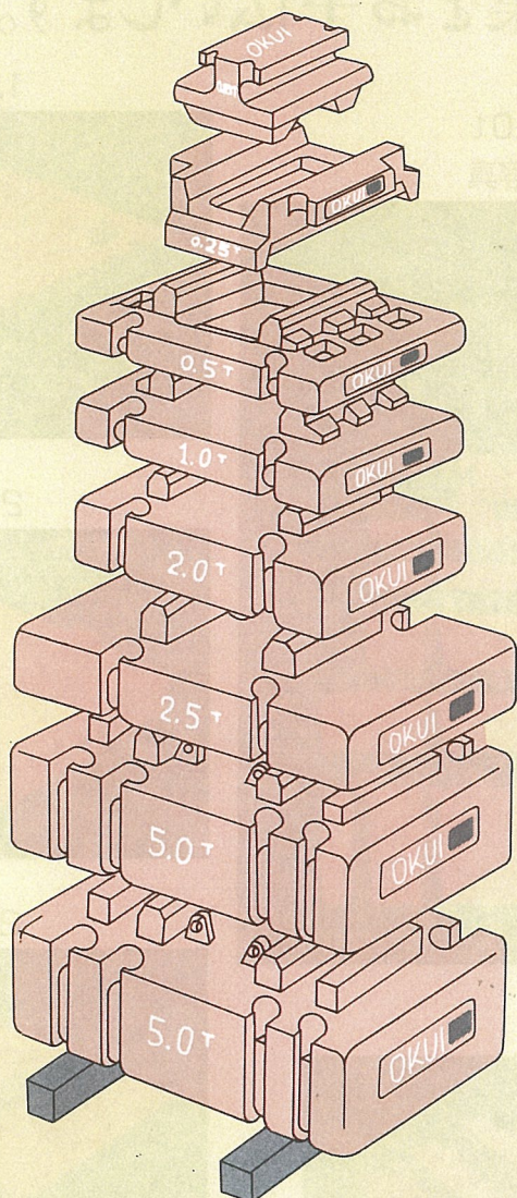
クレーン検査用ウエイト形状寸法
